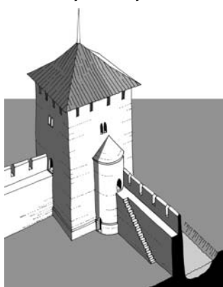
Pokus o rekonstrukci možné podoby hranolové věže se zabudovaným vřetenovitým schodištěm na základě nálezové situace zachycené výzkumem na dvoře fary v roce 2014. (Kresba R. Vrla 2015)
